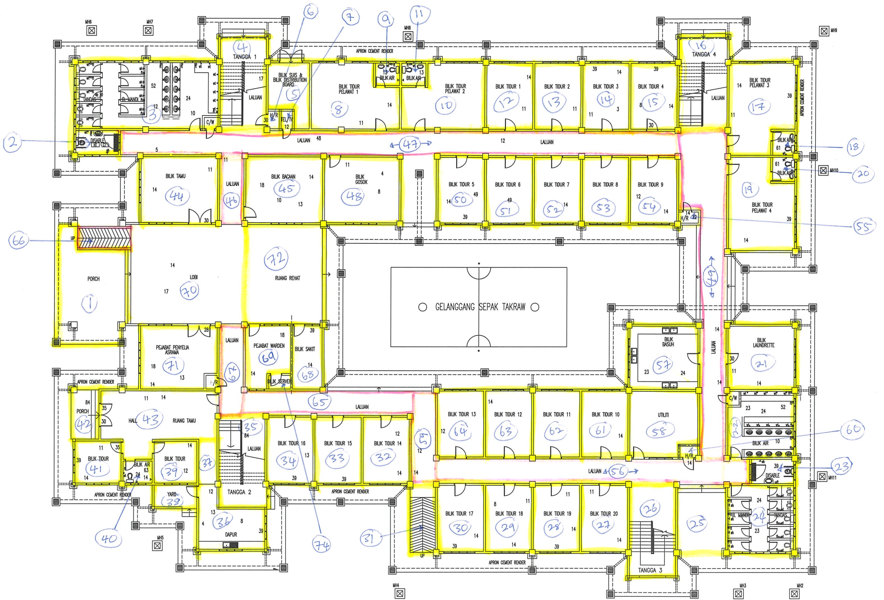
ASRAMA LELAKI A - PELAN LANTAI ARAS TANAH
